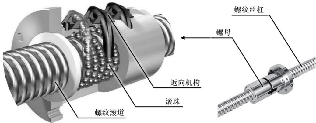
滚珠丝杠副结构示意图
