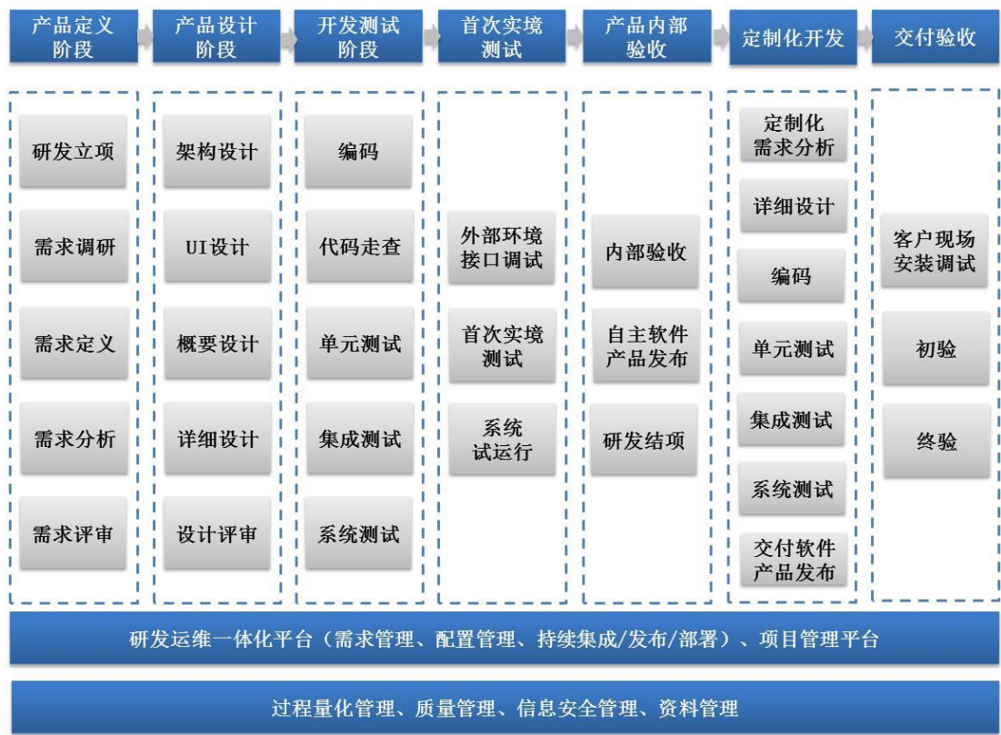
软件开发业务流程示意图
